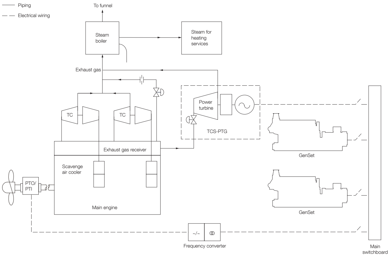
Fig. 4.05.01: PTG diagram
